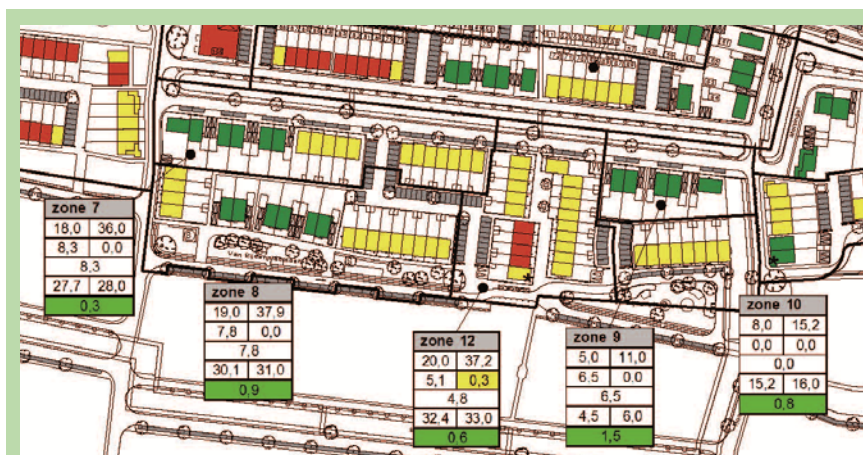
Figuur 3.4 Parkeerbalans Deelgebied 2
